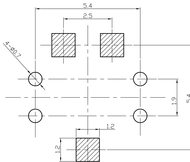
安装尺寸图
