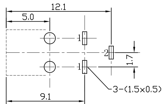
线路板开孔尺寸 P. C. B LAYOUT
