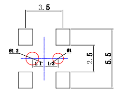
安装尺寸
